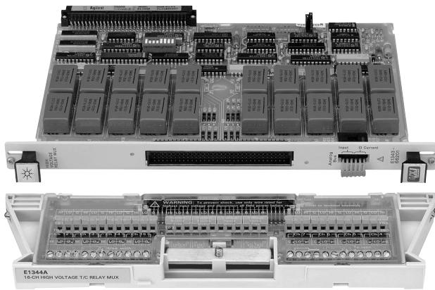
Agilent E1344A
